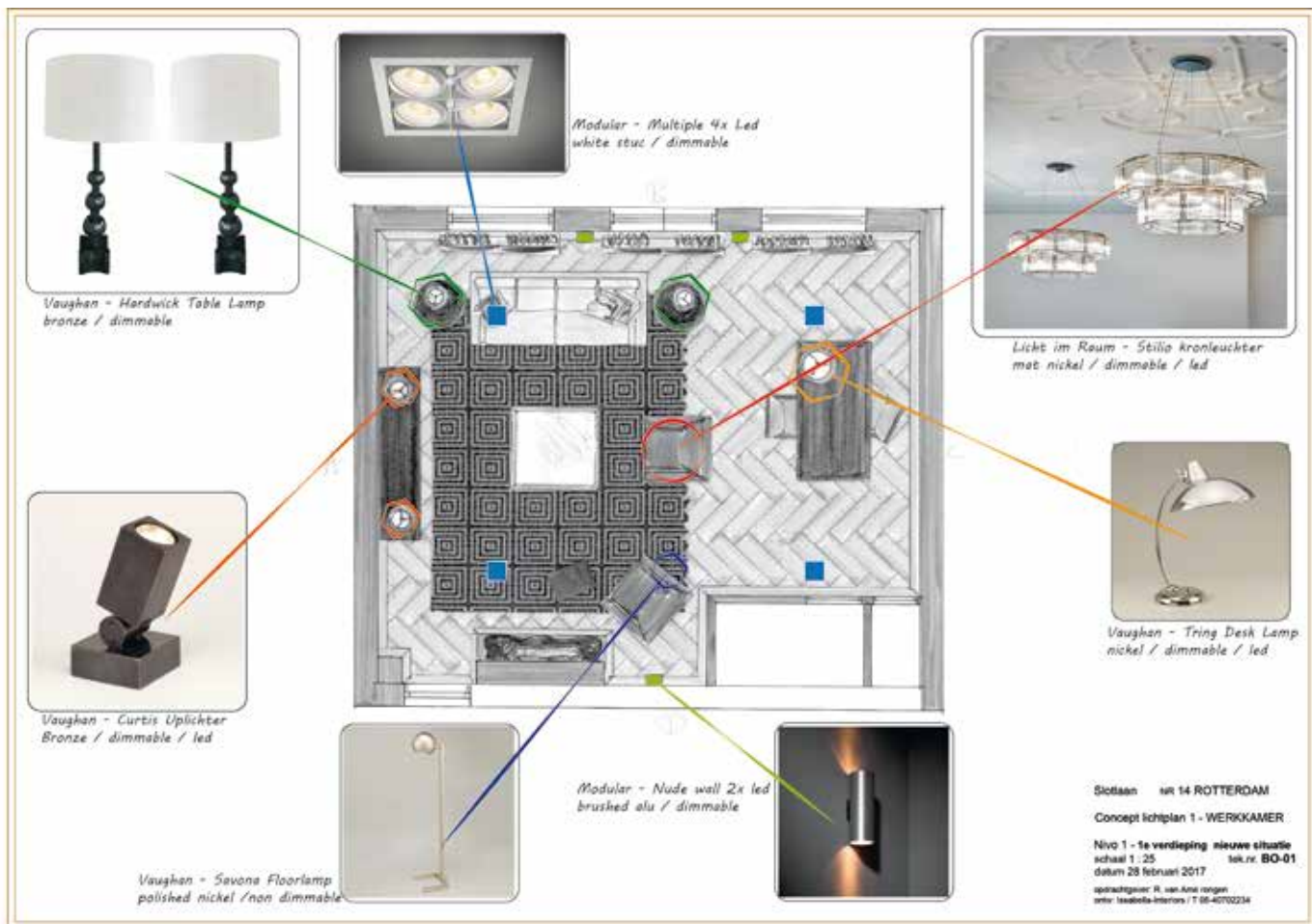
Verlichtingsplan voor een woonhuis in Rotterdam.
